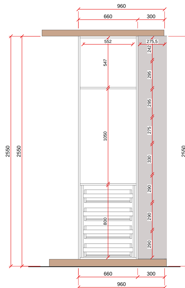
VISTA B - ESC. 1:25
